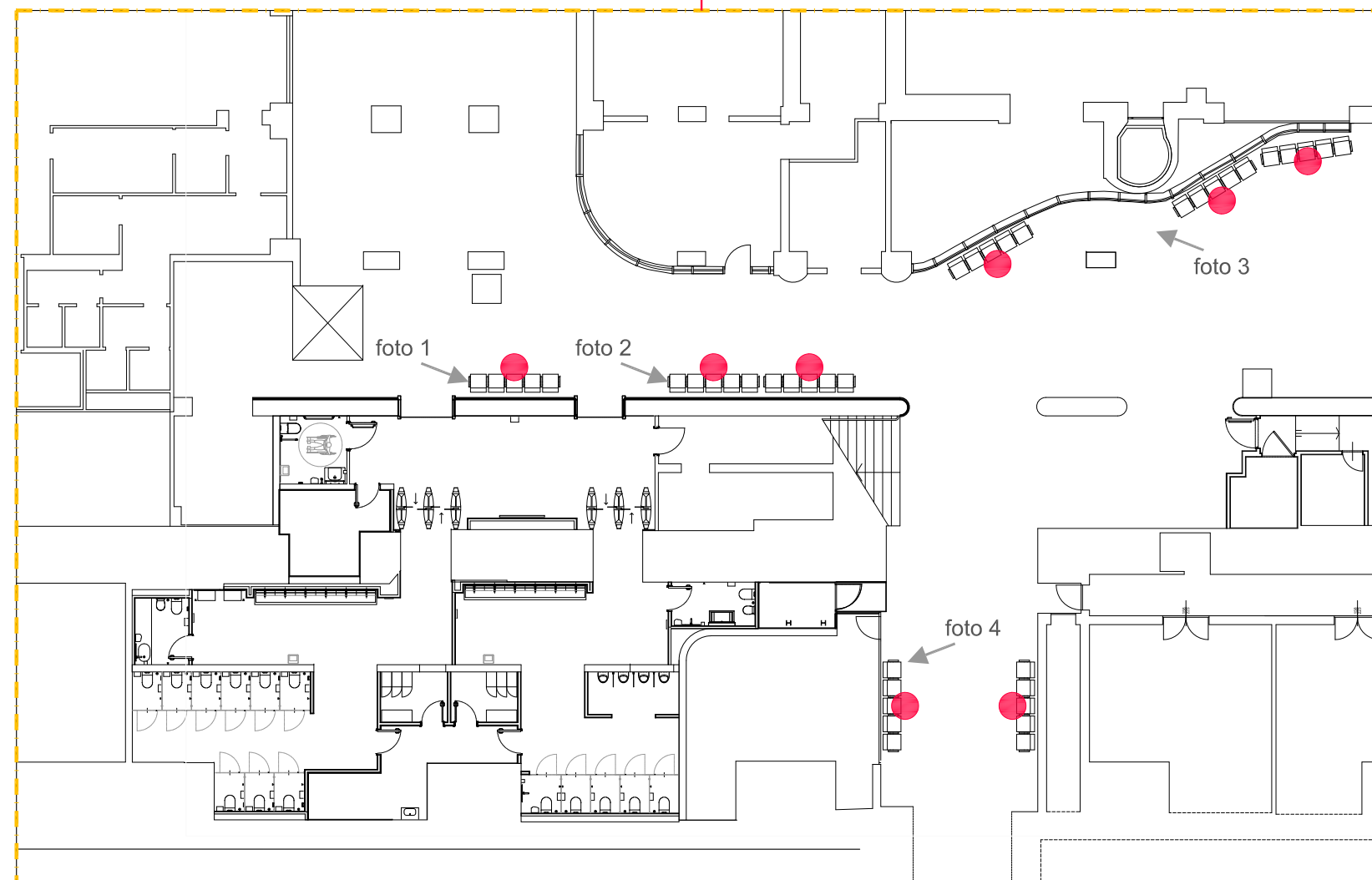
Stralcio Edificio 1 - Piano 1° Interrato (Terra)
