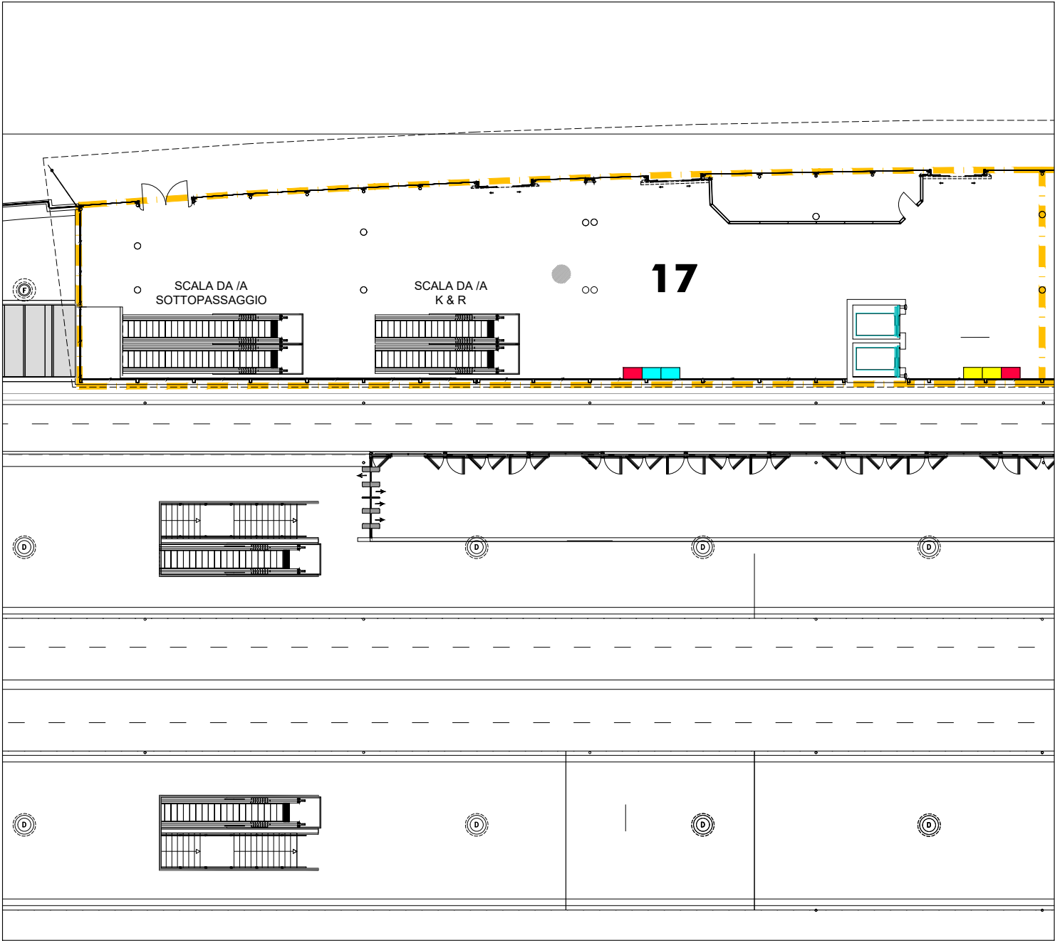
AREA 17
