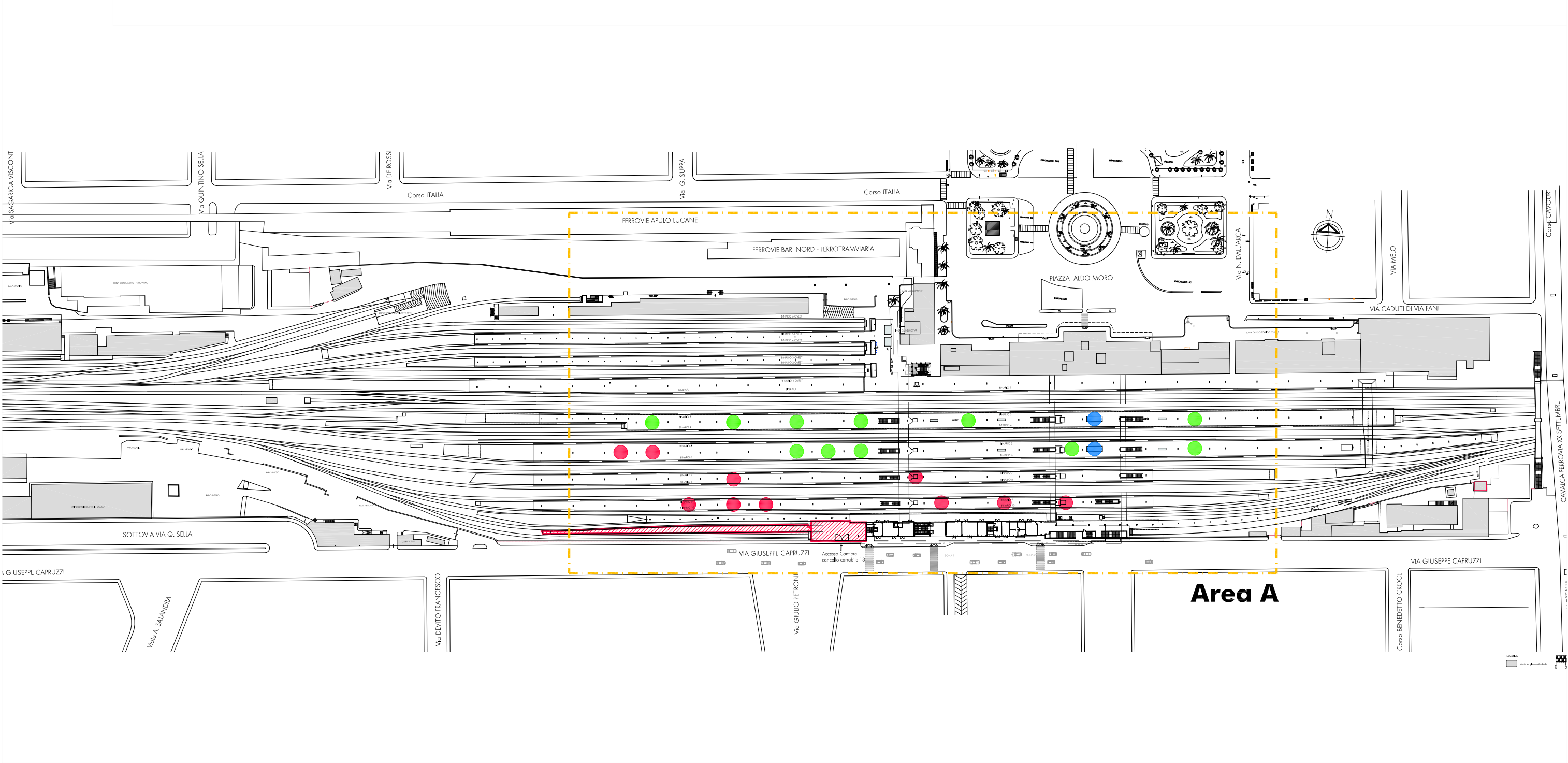
Piano Ferro - Binari
