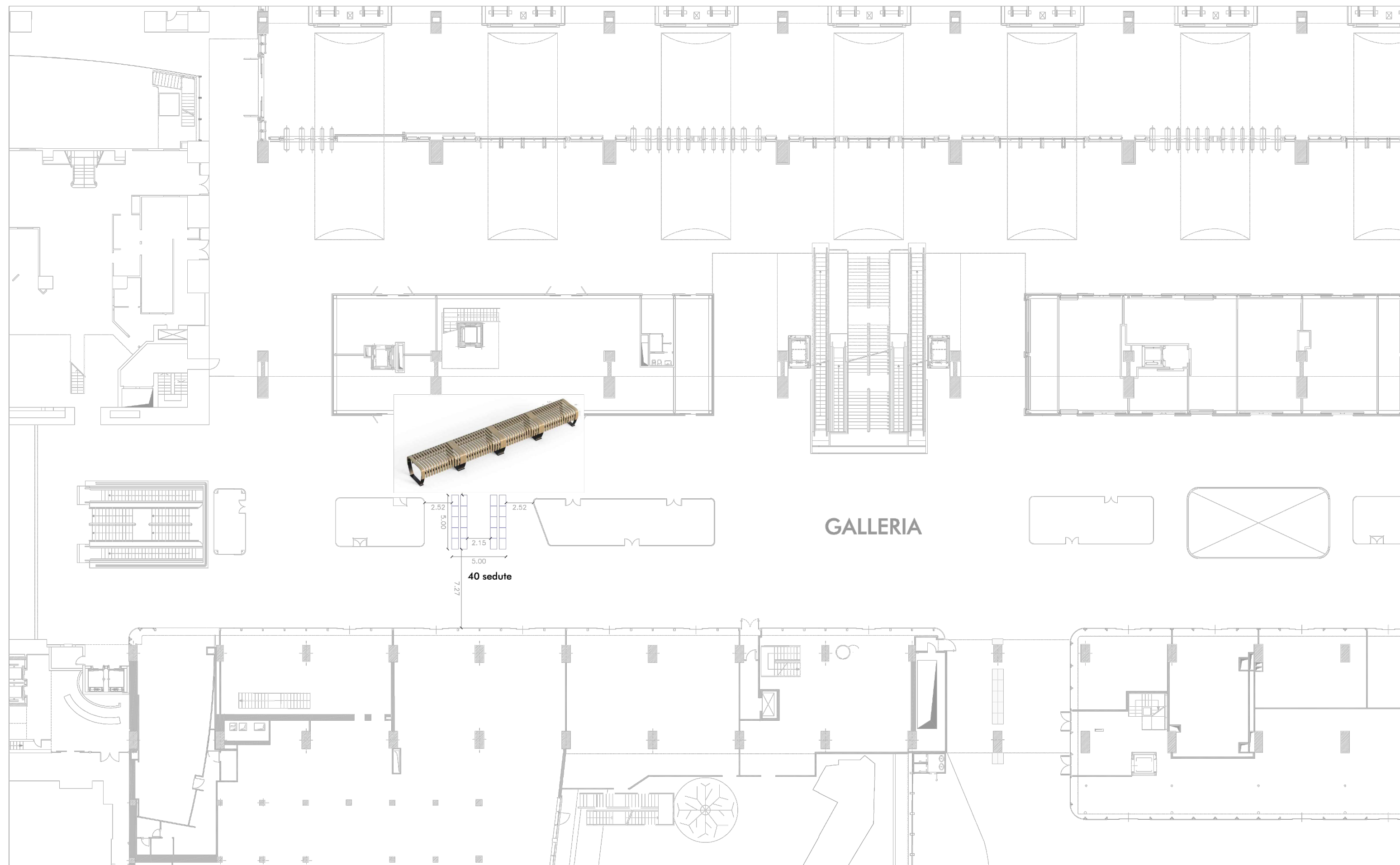
Stazione Roma Termini - Galleria: panche modello GREEN FURNITURE CONCEPT NOVA C BENCH ( 20 moduli da 100 cm = 40 sedute)
