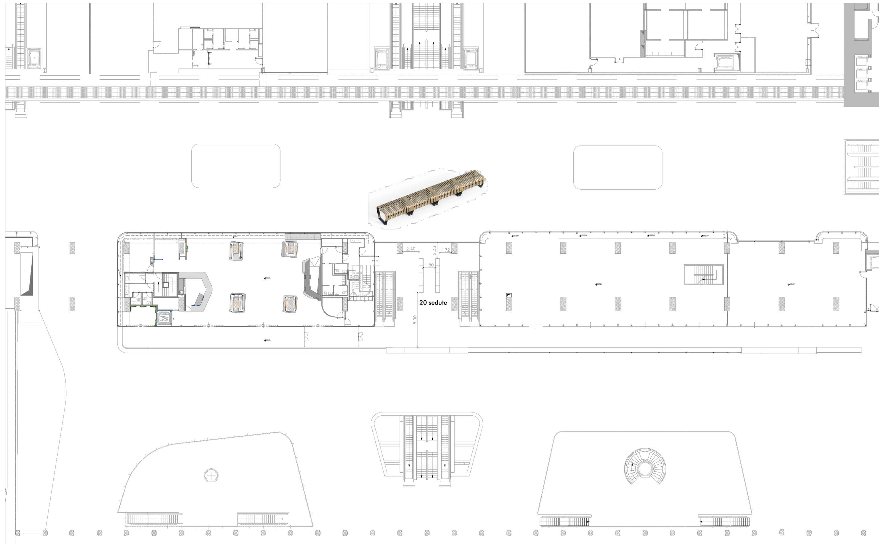
Stazione Roma Termini - Mezzanino: panche modello GREEN FURNITURE CONCEPT NOVA C BENCH ( 10 moduli da 100 cm = 20 sedute )
