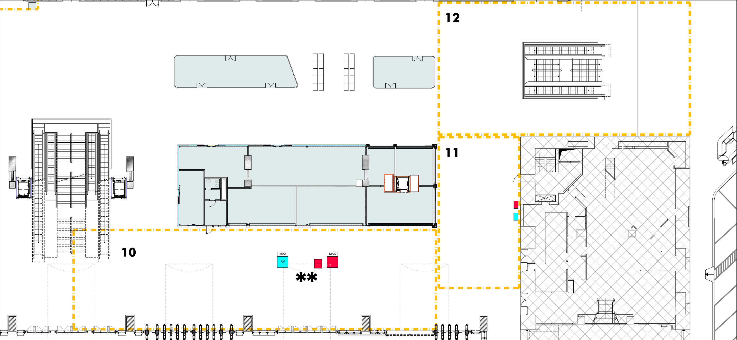
Individuazione Aree ** L'utilizzo dell'area con ingombro MAX è subordinata alla rimozione delle bss presenti Aree 10-11 - Aree Fronte Binari lato Destro / Area 12 - Area Accesso via Marsala
