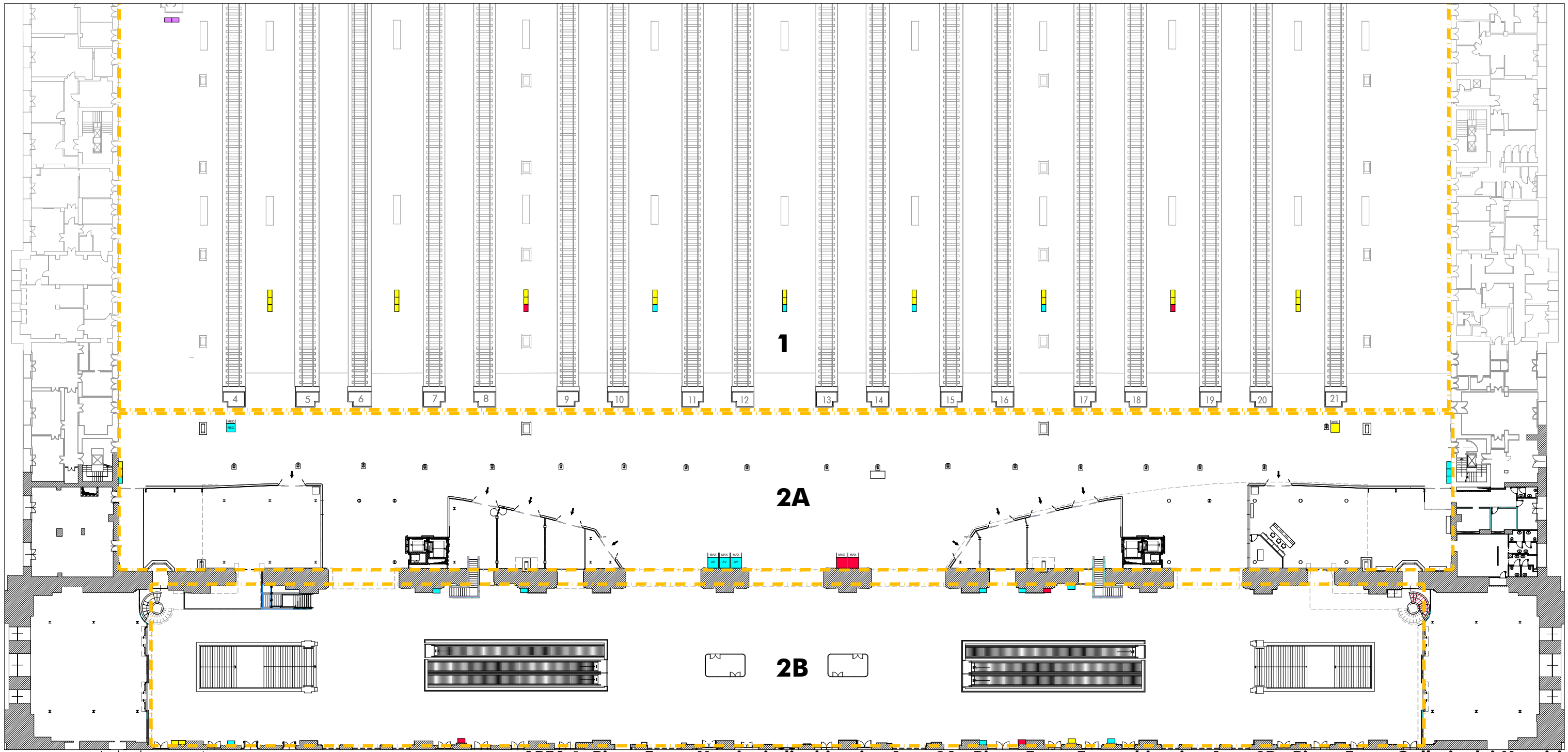
Individuazione Aree AREA 1: Piano Ferro-Marciapiedi e binari Area 2A : Piano Ferro-Fronte binari Area 2B : Piano Ferro-Galleria dei Mosaici MAX Area Desk - Ingombro MAX (200x200x250 – mq max 3,8) MED Area Desk – Ingombro MED (140x120x230) MIN Area Desk – Ingombro MIN (100x50x230)
